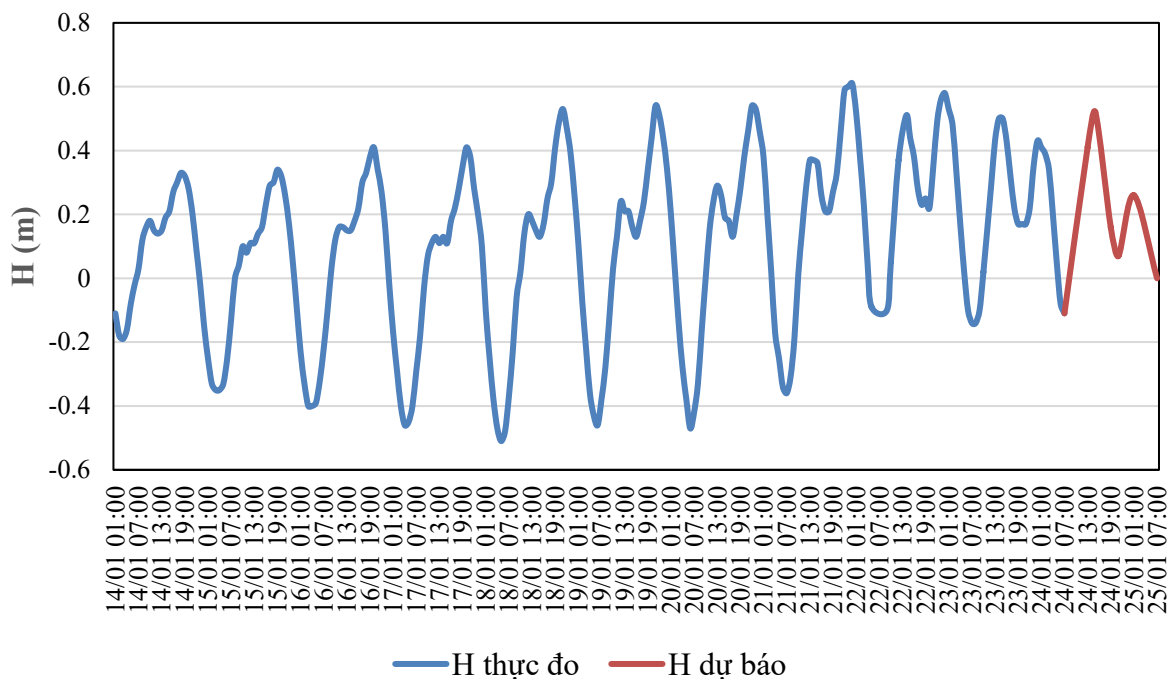
QUÁ TRÌNH MỰC NƯỚC THỰC ĐO VÀ DỰ BÁO TRẠM CẨM LỆ (Từ 01h/14/1 đến 07h/25/1/2026)
