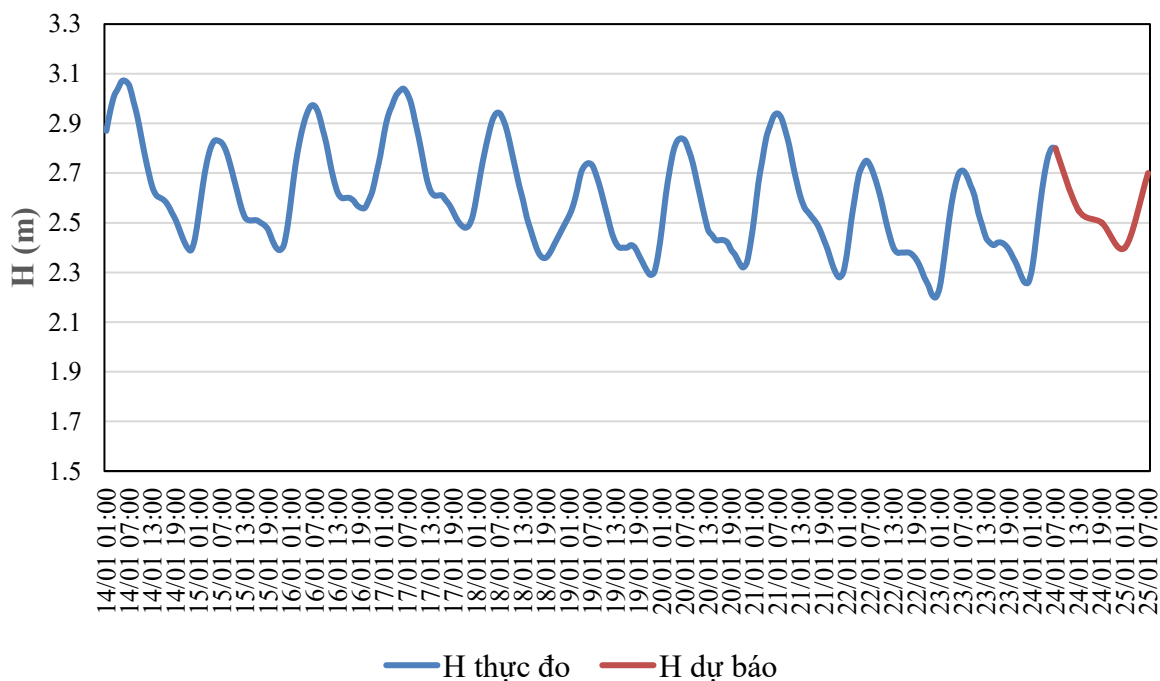
QUÁ TRÌNH MỰC NƯỚC THỰC ĐO VÀ DỰ BÁO TRẠM ÁI NGHĨA (Từ 01h/14/1 đến 07h/25/1/2026)
