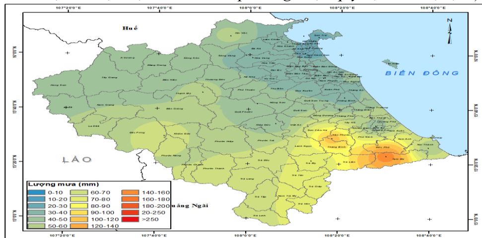
Bản đồ dự báo mưa 24 giờ tới (từ 10h/20/11-10h/21/11) trên đất liền thành phố Đà Nẵng (không bao gồm đặc khu Hoàng Sa)
