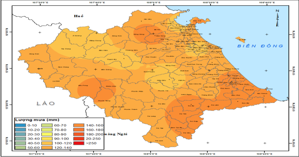
Bản đồ dự báo mưa 24 giờ tới (từ 10h/16/11-10h/17/11) trên đất liền thành phố Đà Nẵng (không bao gồm đặc khu Hoàng Sa)
