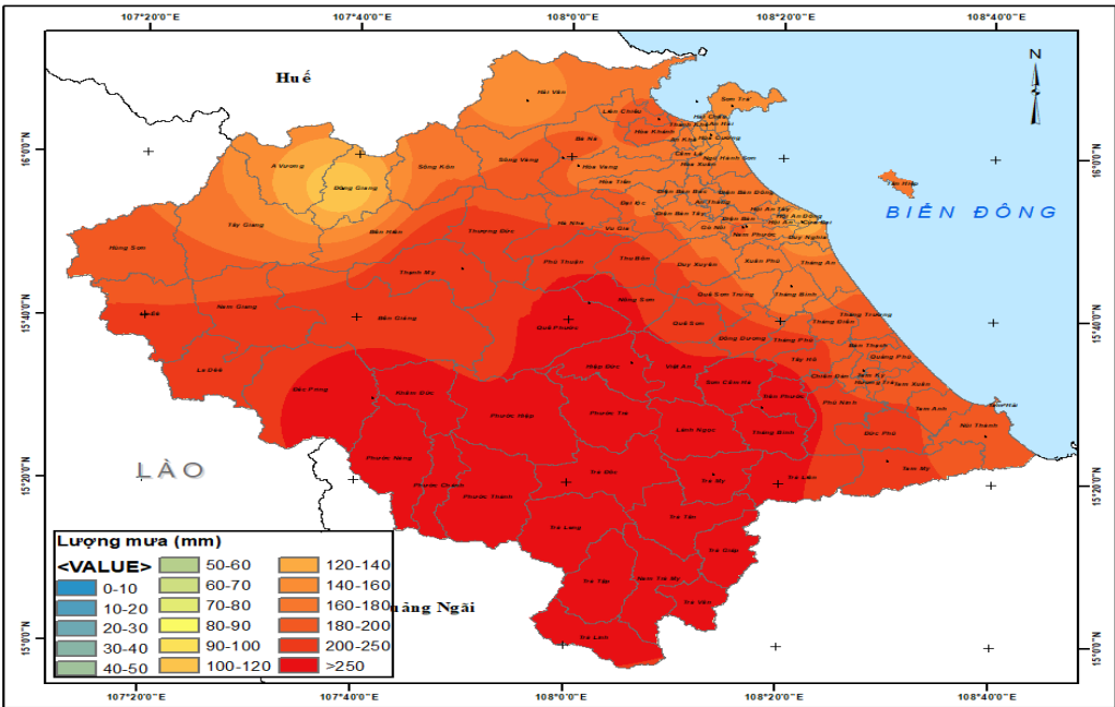
Bản đồ dự báo mưa 24 giờ tới (từ 16h/28/10-16h/29/10) trên đất liền thành phố Đà Nẵng (không bao gồm đặc khu Hoàng Sa)
