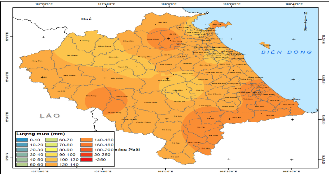
Bản đồ dự báo mưa 24 giờ tới (từ 10h/27/10-10h/28/10) trên đất liền thành phố Đà Nẵng (không bao gồm đặc khu Hoàng Sa)
