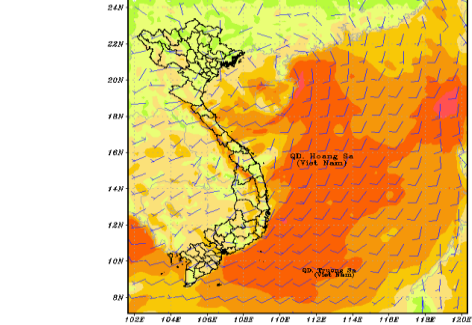
Hướng và tốc độ gió 10m dự báo lúc 22h ngày 25/08/2026
