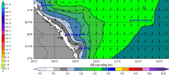
Hình 1: Bản đồ dự báo gió mạnh 24 giờ tới Hình 2: Bản đồ dự báo sóng lớn 24 giờ tới
