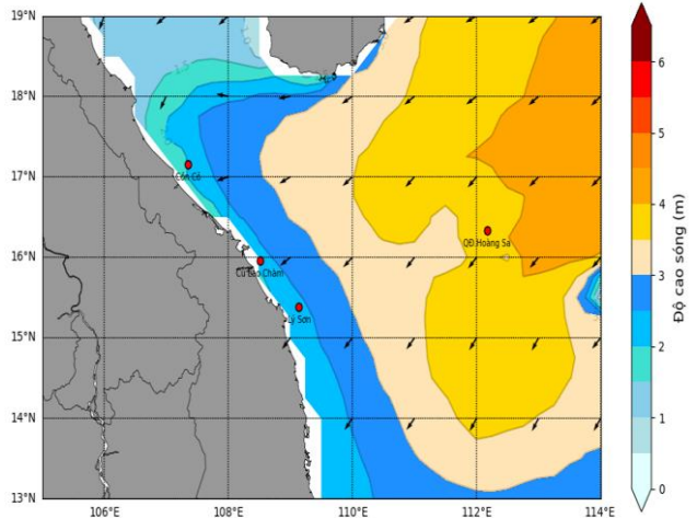
Hình 1: Bản đồ dự báo gió mạnh 24 giờ tới Hình 2: Bản đồ dự báo sóng lớn 24 giờ tới
