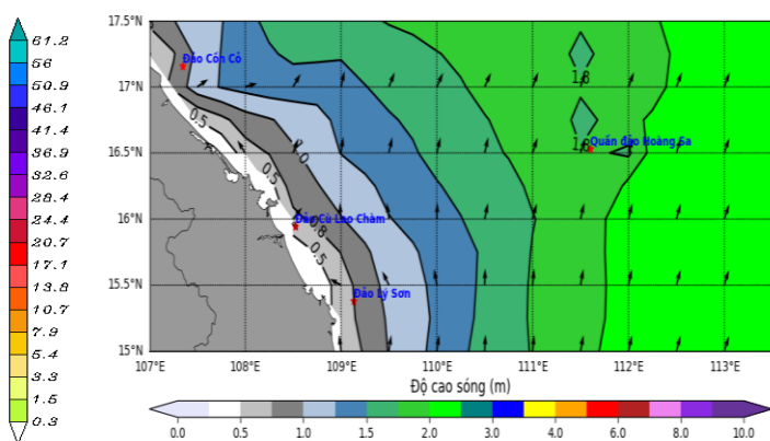
Hình 2: Bản đồ dự báo sóng lớn 24 giờ tới
