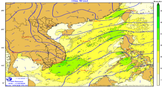
Hình 1: Bản đồ dự báo gió mạnh 24 giờ tới
