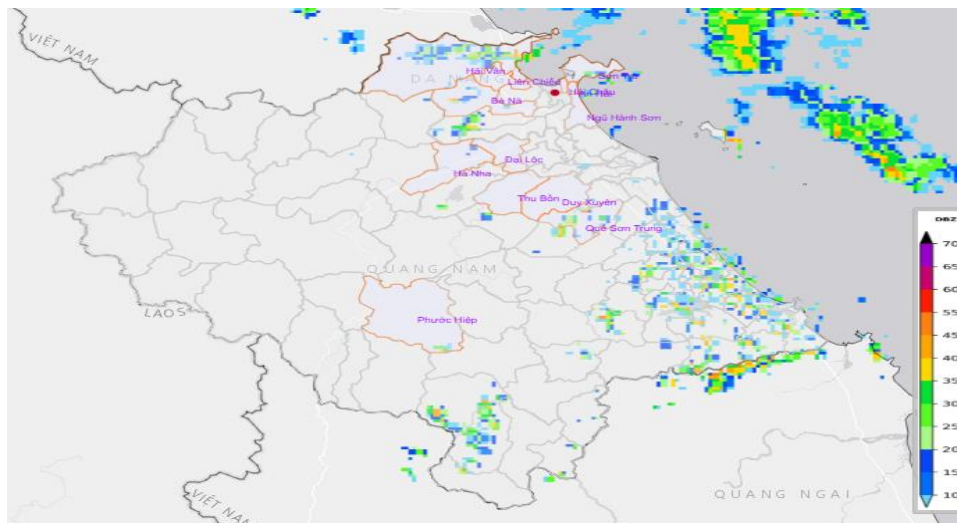
Hình 1: Ảnh ra đa Tam Kỳ lúc 13h00 ngày 19/10/2026 tại TP Đà Nẵng
