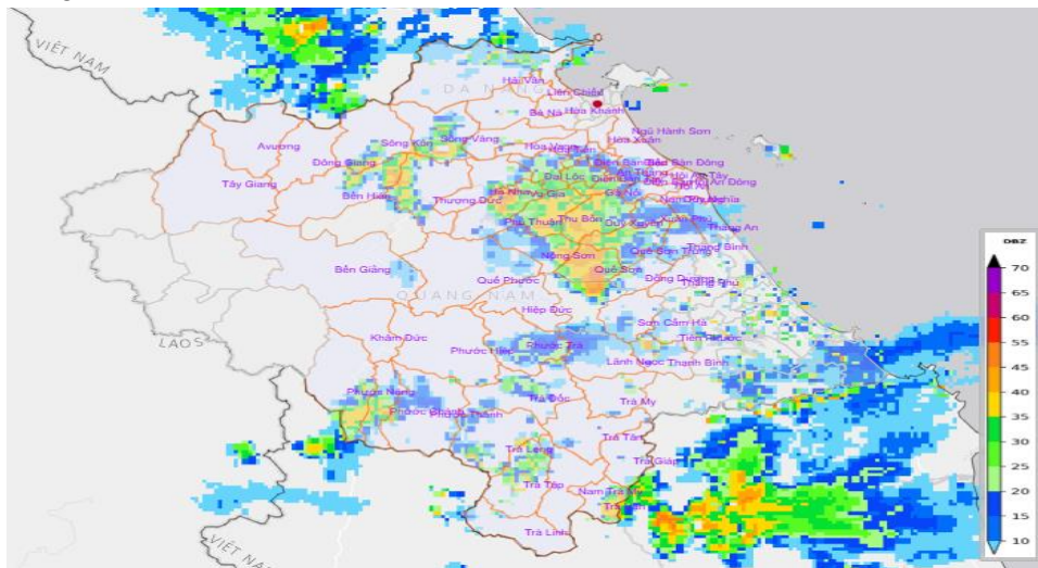
Hình 1: Ảnh ra đa Tam Kỳ lúc 16h10 ngày 27/09/2026 tại TP Đà Nẵng
