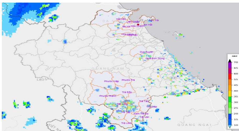
Hình 1: Ảnh ra đa Tam Kỳ lúc 14h50 ngày 16/09/2026 tại TP Đà Nẵng
