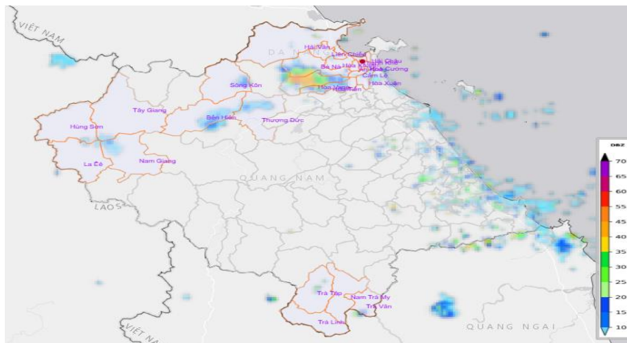
Hình 1: Ảnh ra đa Tam Kỳ lúc 13h40 ngày 11/08/2026 tại TP Đà Nẵng
