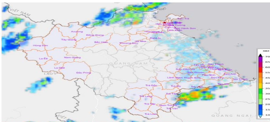
Hình 1: Ảnh ra đa Tam Kỳ lúc 14h20 ngày 02/08/2026 tại TP Đà Nẵng
