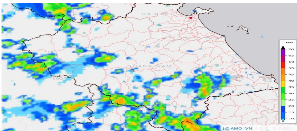
Hình 1: Ảnh ra đa Tam Kỳ lúc 14h10 ngày 30/07/2026 tại TP Đà Nẵng
