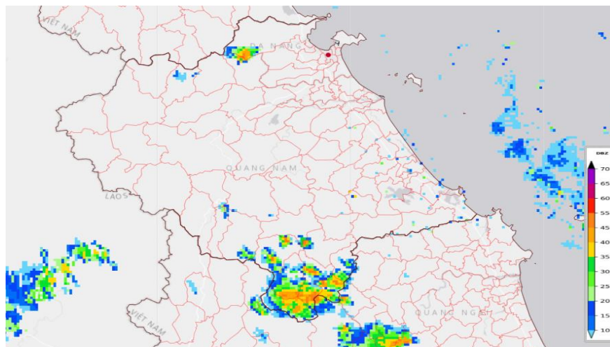
Hình 1: Ảnh ra đa Tam Kỳ lúc 16h10 ngày 22/06/2026 tại TP Đà Nẵng
