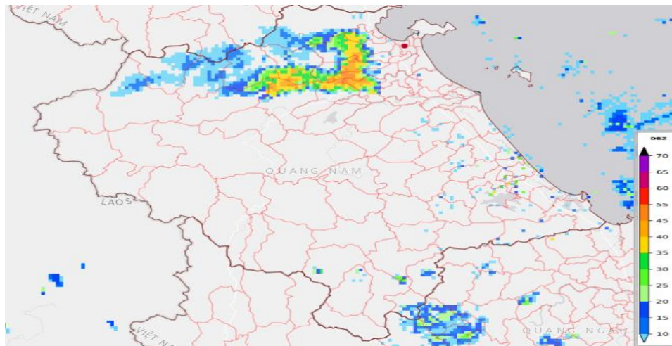
Hình 1: Ảnh ra đa Tam Kỳ lúc 15h00 ngày 16/06/2026 tại TP Đà Nẵng
