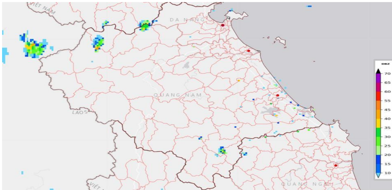
Hình 1: Ảnh ra đa Tam Kỳ lúc 15h50 ngày 01/06/2026
