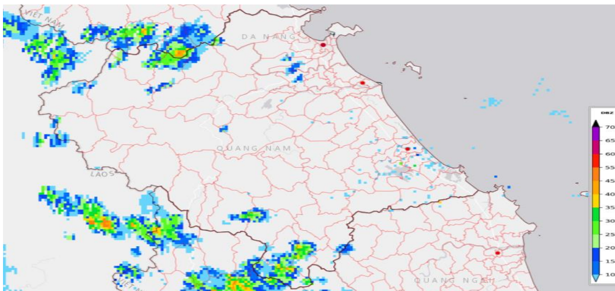
Hình 1: Ảnh ra đa Tam Kỳ lúc 14h00 ngày 26/04/2026
