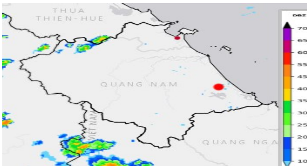
Hình 1: Ảnh ra đa Tam Kỳ lúc 15h10 ngày 01/10/2025
