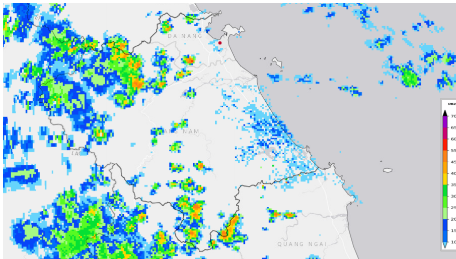
Hình 1: Ảnh ra đa Tam Kỳ lúc 13h00 ngày 07/09/2025
