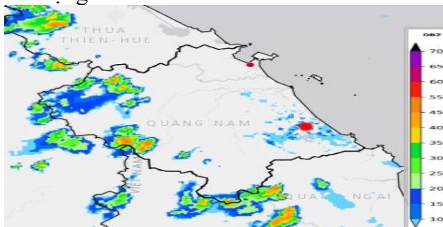
Hình 1: Ảnh ra đa Tam Kỳ lúc 15h20 ngày 23/8/2025
