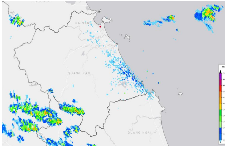
Hình 1: Ảnh ra đa Tam Kỳ lúc 13h50 ngày 21/8/2025
