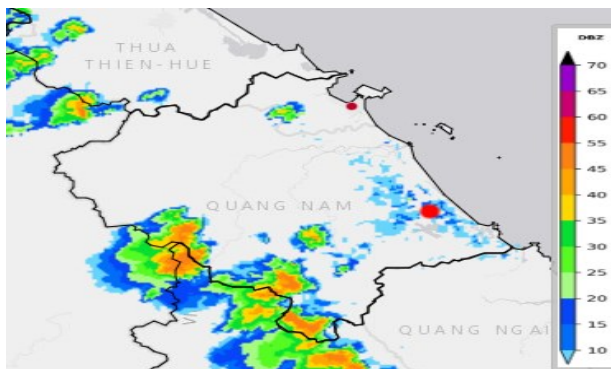
Hình 1: Ảnh ra đa Tam Kỳ lúc 15h10 ngày 20/8/2025
