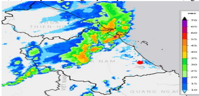
Hình 1: Ảnh ra đa Tam Kỳ lúc 16h00 ngày 18/8/2025
