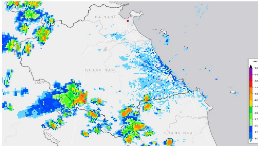
Hình 1: Ảnh ra đa Tam Kỳ lúc 14h20 ngày 07/8/2025
