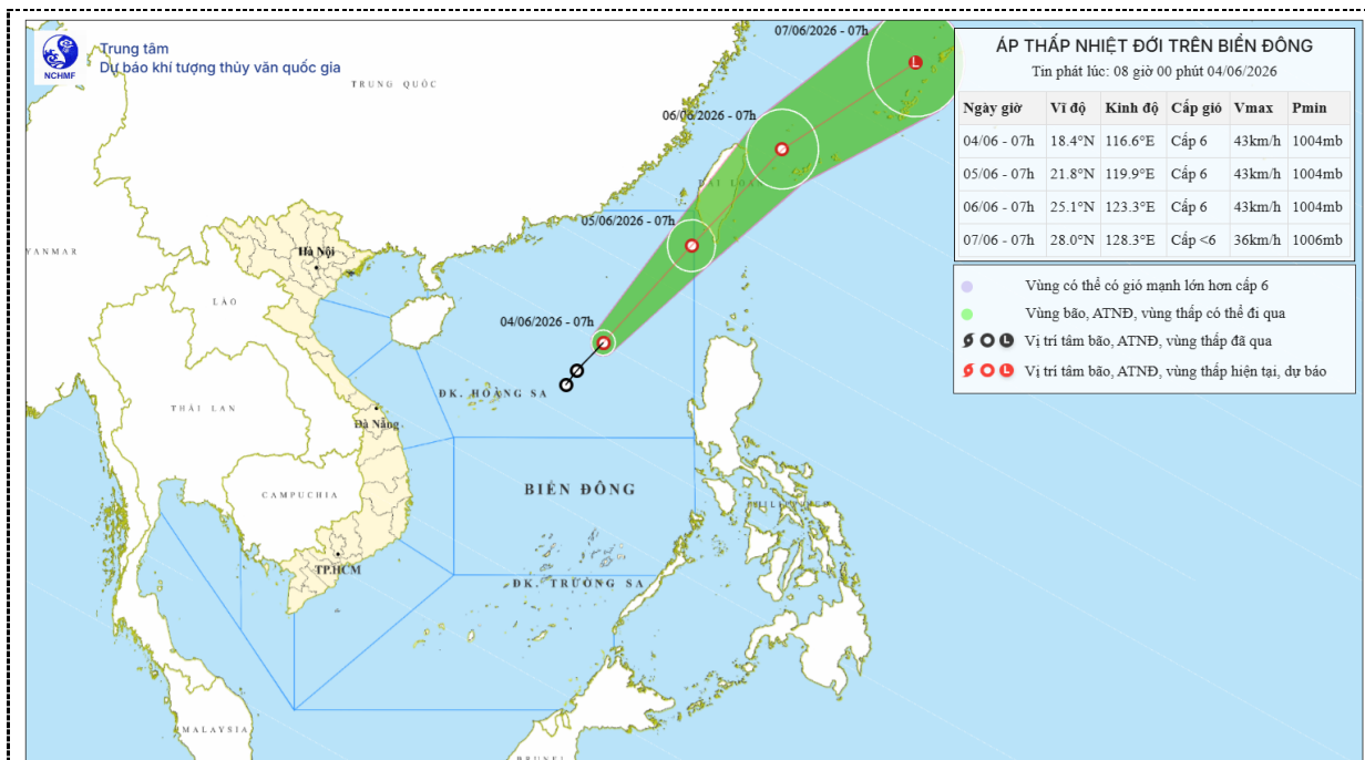
Hình1. Bản đồ dự báo quỹ đạo và cường độ áp thấp nhiệt đới lúc 08h00 ngày 04/6/2026
