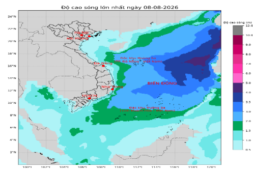
Hình 2. Bản đồ dự báo độ cao sóng
