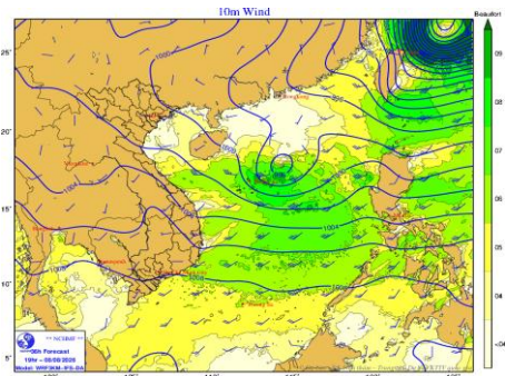
Hình 1. Bản đồ dự báo gió mạnh
