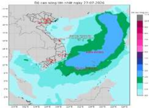
Hình 2. Bản đồ dự báo độ cao sóng
