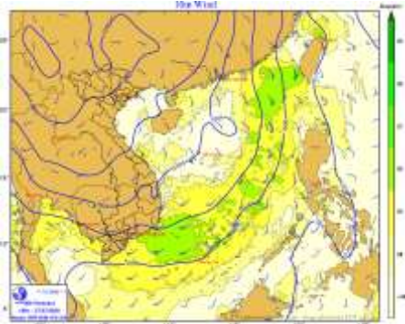
Hình 1. Bản đồ dự báo gió mạnh
