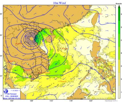
Hình 1. Bản đồ dự báo gió mạnh
