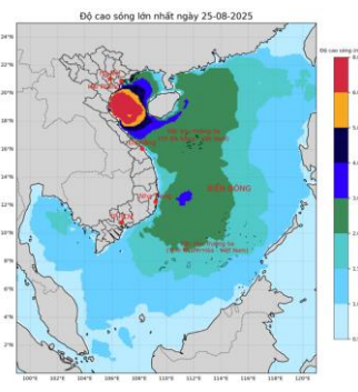
Hình 2. Bản đồ dự báo độ cao sóng
