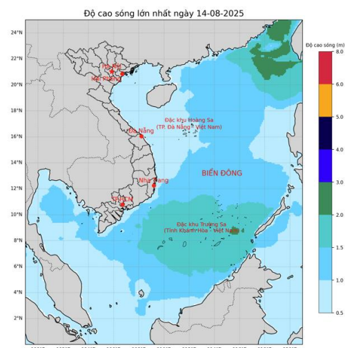
Hình 2. Bản đồ dự báo độ cao sóng
