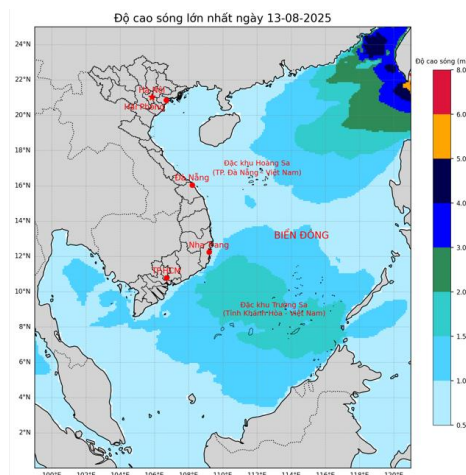
Hình 2. Bản đồ dự báo độ cao sóng
