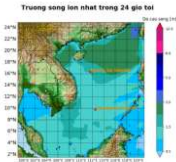
Hình 2. Bản đồ dự báo độ cao sóng
