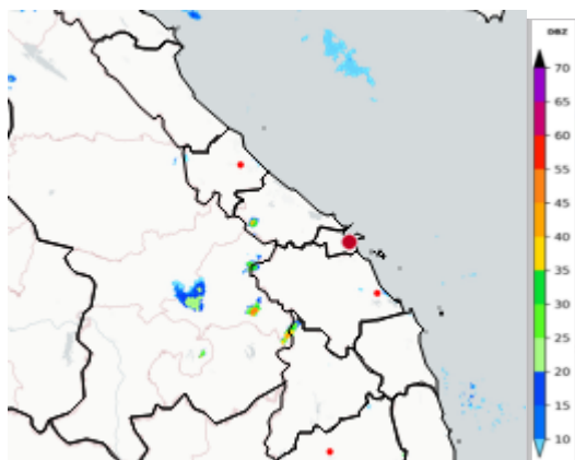
Hình 1: Ảnh ra đa thời tiết tại khu vực Trung Trung Bộ
